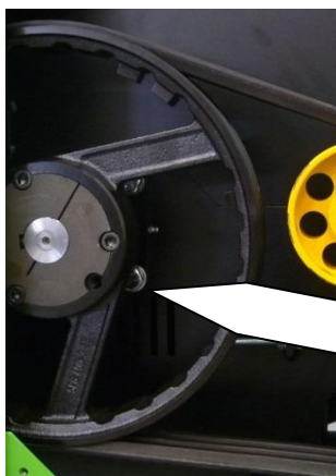
Anbringung des Drehzahlgebers unter der Haube
