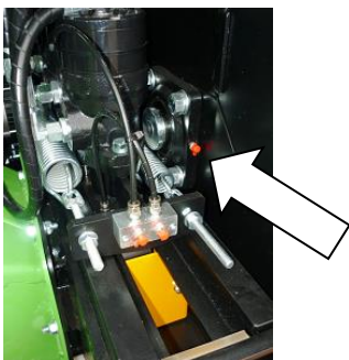
Schmierbüchsen an Lagerung der Zerkleinerungsscheibe
