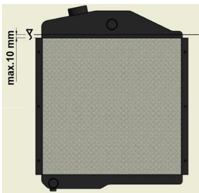
Deckel öffnen und Kühlflüssigkeit einfüllen.
