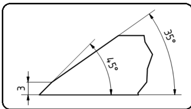
Schneidegeometrie der Messerschneide
